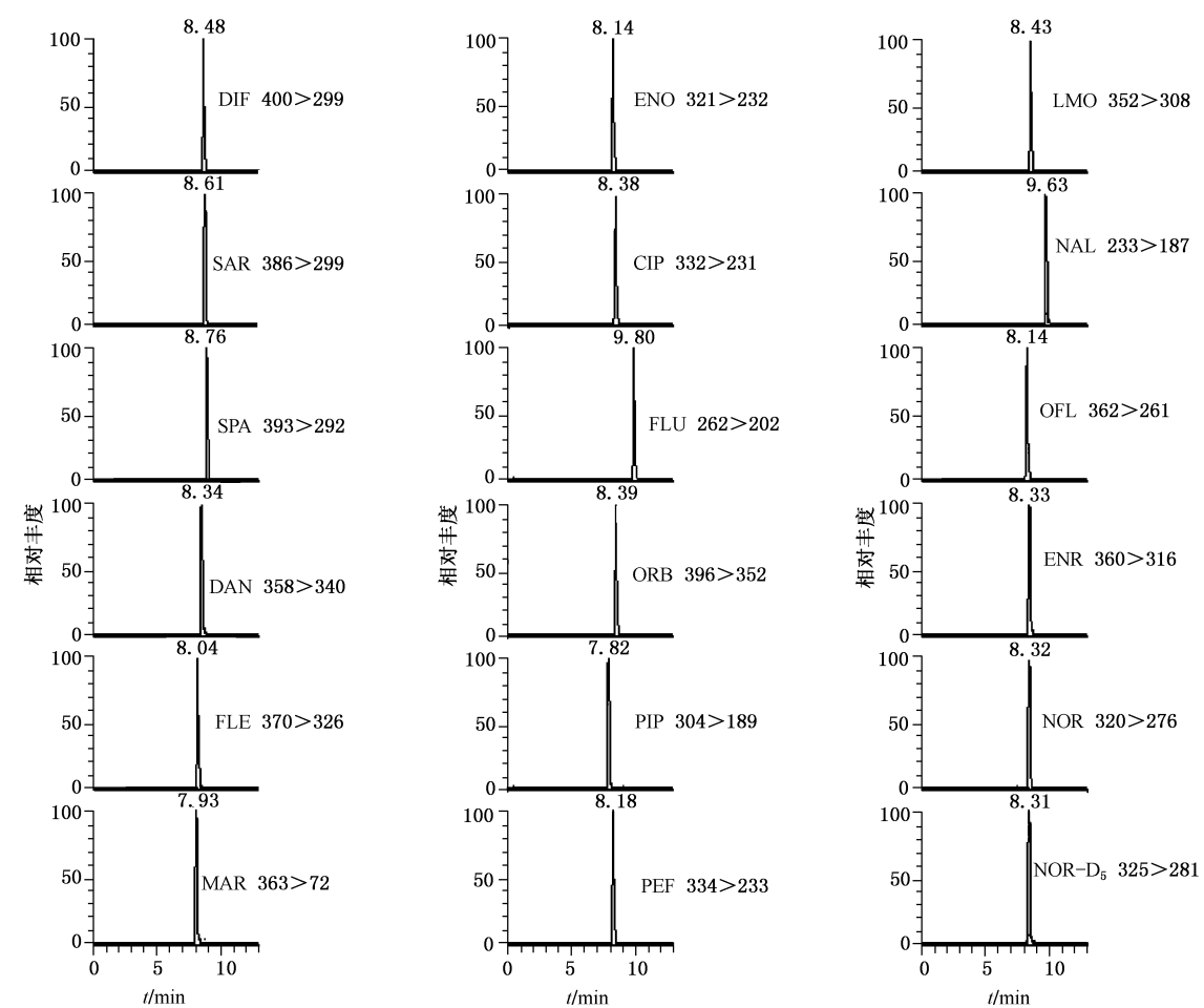
图 D.1 喹诺酮类药物及其内标离子流色谱图
